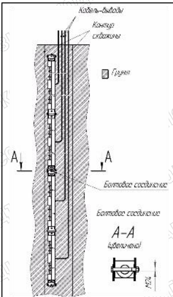
Установка АЗЖК-РА-ГС в грунт без магистрального кабеля
